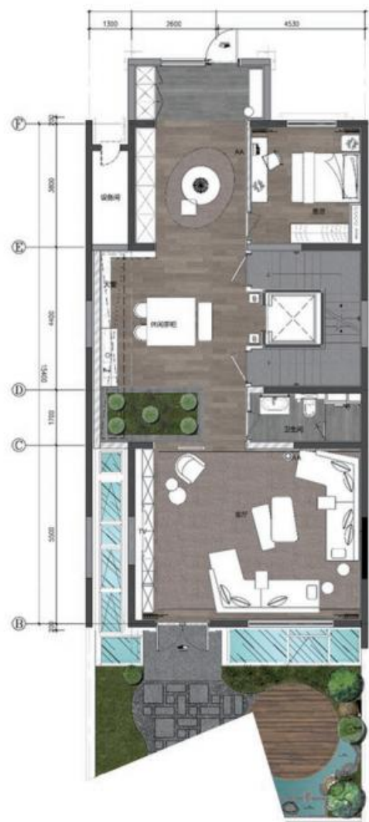
一层平面图
