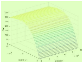
图 13 不同阻尼系数下的功率分布图
