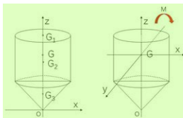
图 11 重心位置确定 5
