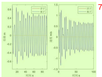
图 3 题 1.(1) 大地坐标系下浮子和振子的垂荡位移和速度 8
