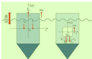
图2 垂荡运动受力分析示意图
