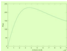
图7 题 2.(1) 直线阻尼系数与平均输出功率的关系
