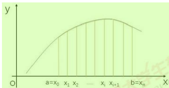
图 6 梯形法求积分
