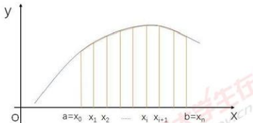
图 6 梯形法求积分
