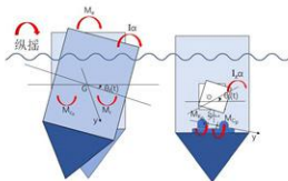
图 10 纵摇运动受力分析示意图
