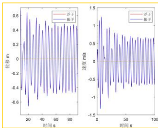
图 3 题 1.1 大地坐标系下浮子和振子的垂荡位移和速度
