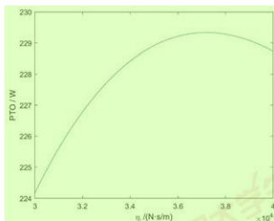
图 4 PTO 关于 \eta_l 的函数图 2
