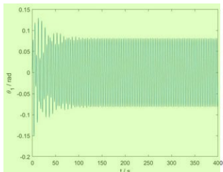
图 10 \theta_1 关于时间的变化
