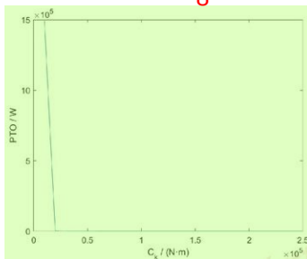
图 17 扭转弹簧刚度的稳定性分析图
