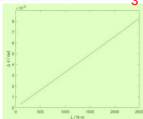
图 16 波浪激励力矩的稳定性分析图
