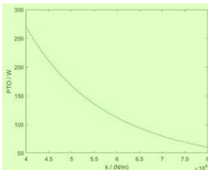
图 18 弹簧刚度的稳定性分析图
