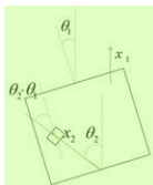
图 9 以中轴与底座连接转轴 O 建立平动非惯性系
