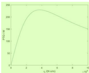
图 3 PTO 关于 \eta_l 的函数图 1
