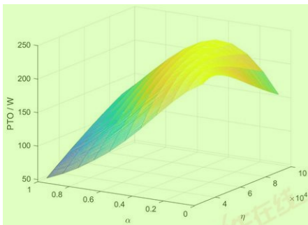
图 5 PTO 关于比例系数 \eta 和幂指数 \alpha 的函数图
