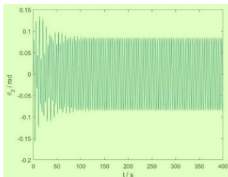
图 11 \theta_2 关于时间的变化
