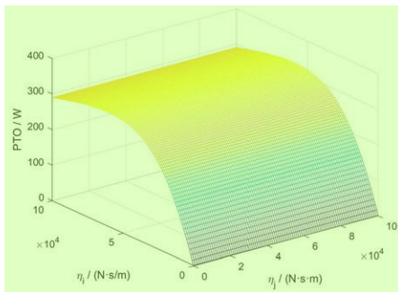
图 12 PTO 关于 \eta_i 和 \eta_j 的全局遍历图
