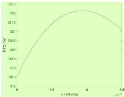
图 13 PTO 关于 \eta_l 的局部遍历图
