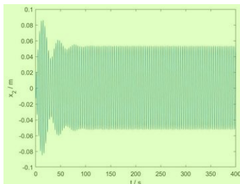
图 8 x_2 关于时间的变化
