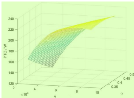
图 6 PTO 关于比例系数 \eta 和幂指数 \alpha 的函数图
