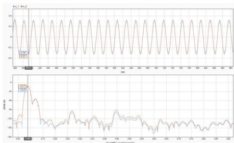
图 14 频率分析
