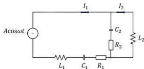
图 6 力电比拟等效电路图
