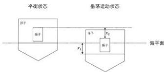
图1 浮子坐标示意图
