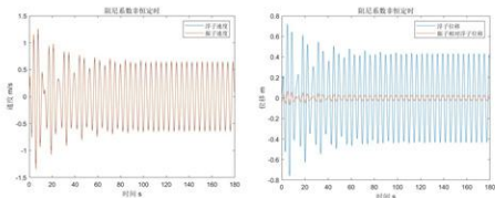
图 5 阻尼系数非恒定时结果曲线
