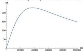
图 7 P_2 关于 R_2 的函数图像
