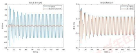
图4 阻尼系数恒定时结果曲线
