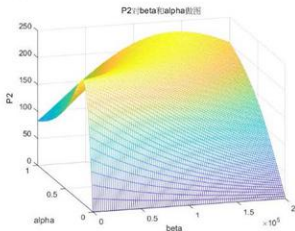
图 8 P 对 \beta 和 \alpha 作图
