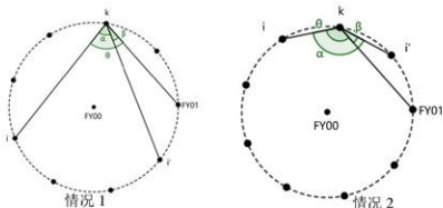
图 6-2 无人机 i 与无人机 i' 的关系图
