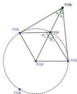
图 7-3 长度坐标调整示意图
