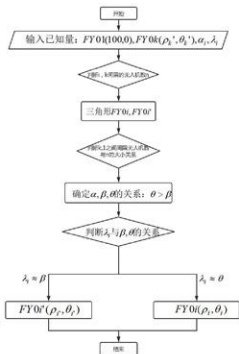
图 6-3 求解流程图
