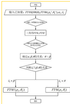
图 6-3 求解流程图
