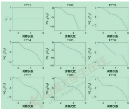
图 16: 不同无人机与标准位置的距离随调整次数的变化
