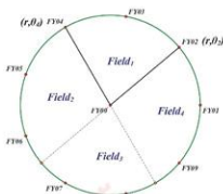
图 3: 正弦定理求解坐标的局限性
