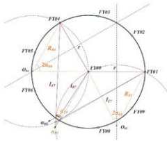
图 4: 等角对等边示意图
