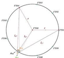
图 1: 三架无人机无源定位示意图
