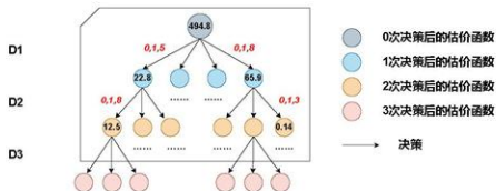
图 14: 决策树示意图
