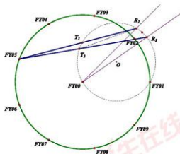
图 11: 角度误差证明示意图
