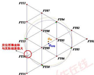
图 17: 四点共圆情况示意
