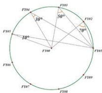
图 6: 标准位置角度 (1)
