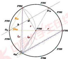
图 5: 圆心坐标的求解
