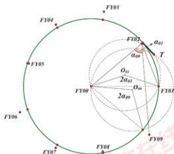
图 13: 确定初始点坐标
