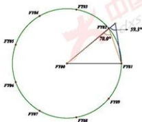
图 9: 误差过大示意图
