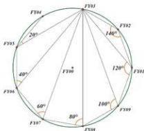
图 7: 标准位置角度 (2)
