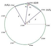
图 2: 正弦定理求解坐标
