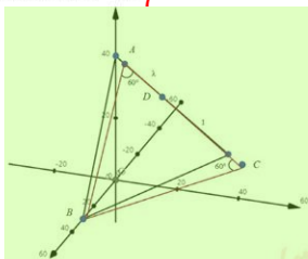
图 21 引理 2 的几何关系
