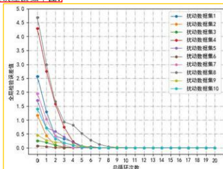
图 28 十组数据集的全局检验误差值
