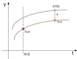
图 3 预测示意图
