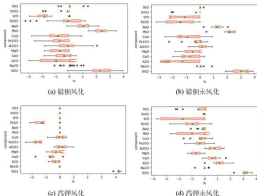
图 1 四类箱线图
