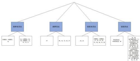
图 7 亚分类结果
