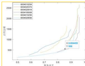
图 5：占用资金随服务水平变化
