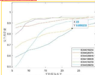
图 4: 平均服务水平随安全库存量的变化
