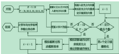
图5 算法1的流程图
