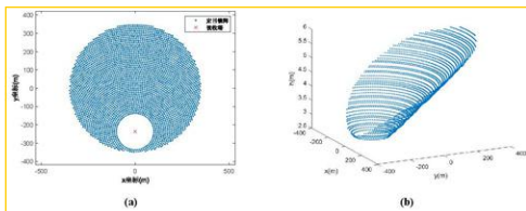
图9 调节后定日镜场中定日镜排布图
