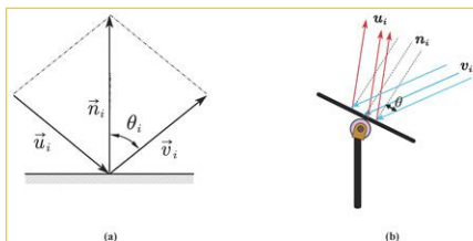
图 3 各方向向量、法向量、反射角图示
