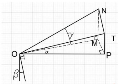
图 3 关于非斜坡角的线面角的示意图
