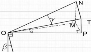
图 3 关于非斜坡角的线面角的示意图
