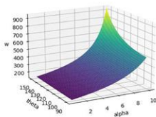
图 18 不同张角和坡度下最大覆宽变化图
