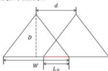
图 1 水平状态下重叠率的定义
