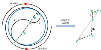
图12. 调头区域圆弧分析图
