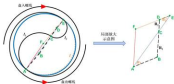
图13.辅助线分析示意图
