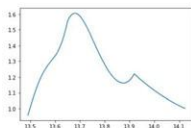
图 4.29: 龙头进入盘出螺线过程中, 第三节龙身前把手的速度
