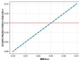
图15 dis(t) 最小值随螺距 d 变化图像
