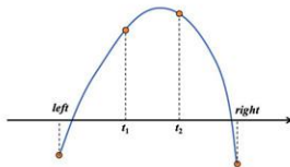
图 21 三分搜索法示意图
