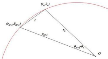
图 2 相邻把手几何关系示意图
