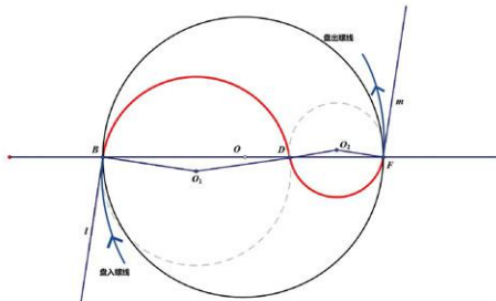
图 16 调头曲线示意图
