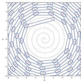
图8 停止盘入时刻板凳龙碰撞情况
