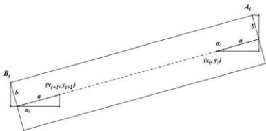
图 6 编号为 i 的板凳几何关系示意图
