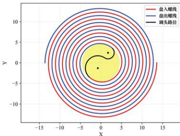
图 18 板凳龙调头路径示意图
