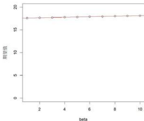
图3 \beta 变动对期望影响表
