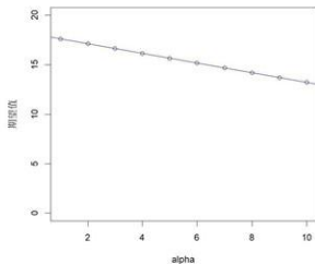
图2 \alpha 变动对期望影响表
