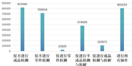
图 12 最优决策与其他决策对比图
