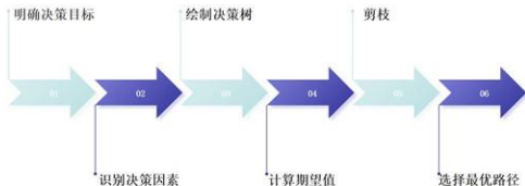
图3 决策树法的一般步骤流程图
