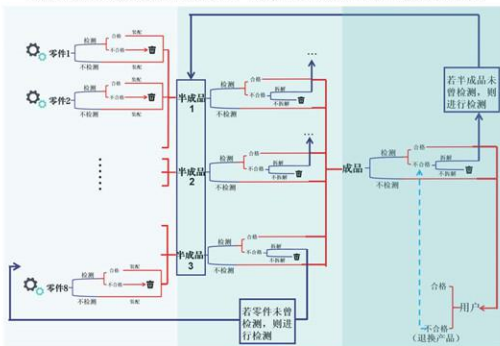
图 7 问题三决策树法分析流程图
