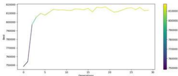
图 10 每代最优个体变化图
