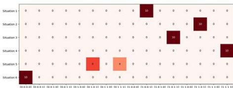
图 14 问题二 95%信度下最优决策分布
