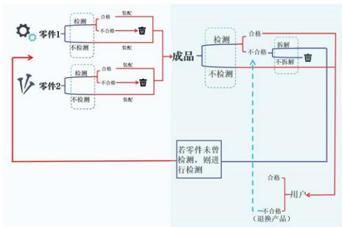
图 4 问题二决策树法分析流程图
