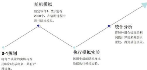
图5 蒙特卡洛算法的步骤具体实现
