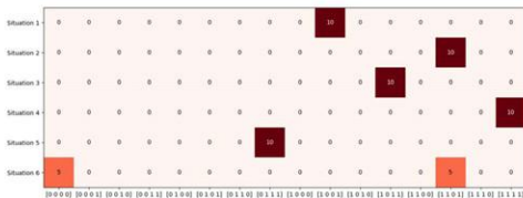
图 15 问题二 90%信度下最优决策分布
