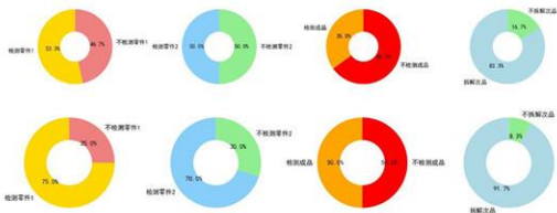
图 16 原决策与 90%信度下 60 种最优决策选择率对比 从图中可以看出，检测决策的选择率均有提升，但由于成品的检测成本高，部分
