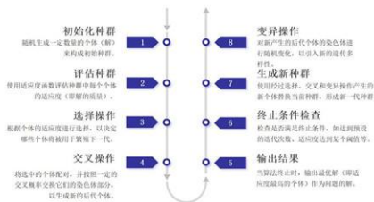
图8 遗传算法的具体步骤
