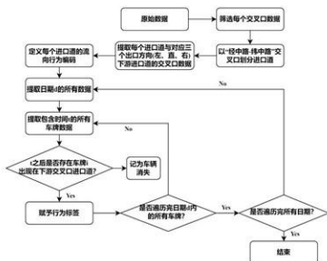
图 4 交叉口流量转向识别方法
