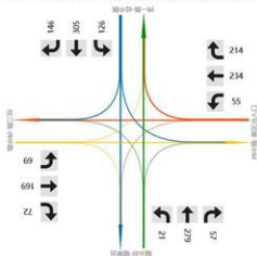
图 5 经中路-纬中路交叉口流量流向图
