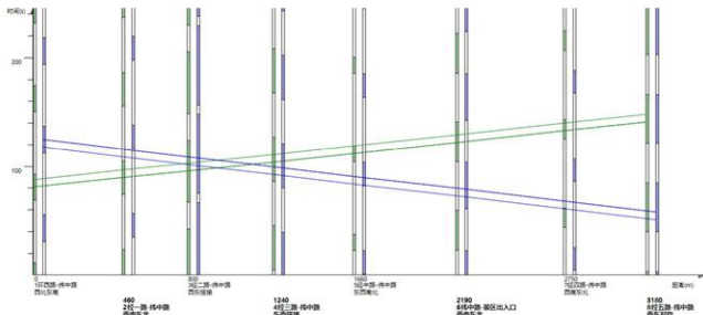
图 6 各交叉口时距图
