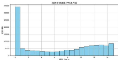
图 4 巡游车辆速度分布直方图
