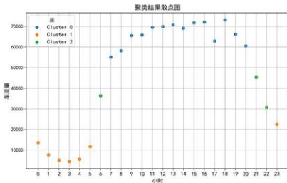
图 3 聚类结果散点图
