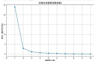
图 2 肘部法求解最佳聚类数 k
