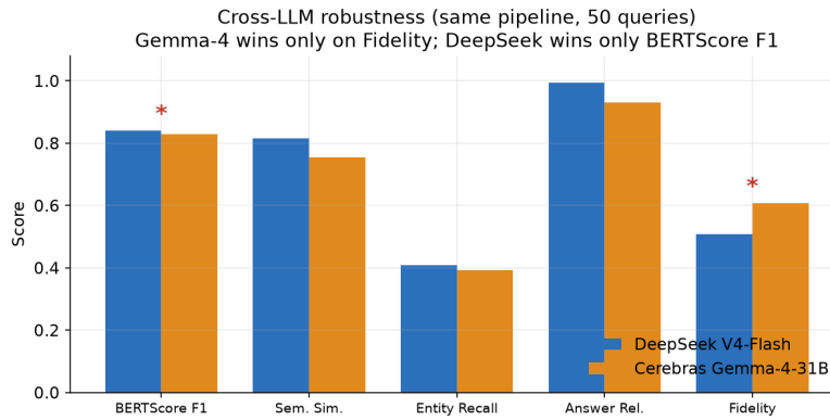
Figura 4. Robustez ante el cambio de generador: Gemma-4 solo gana en Fidelidad; DeepSeek solo gana en BERTScore F1.
