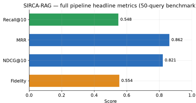
Figura 2. Métricas principales del pipeline completo sobre el benchmark de 50 consultas.
