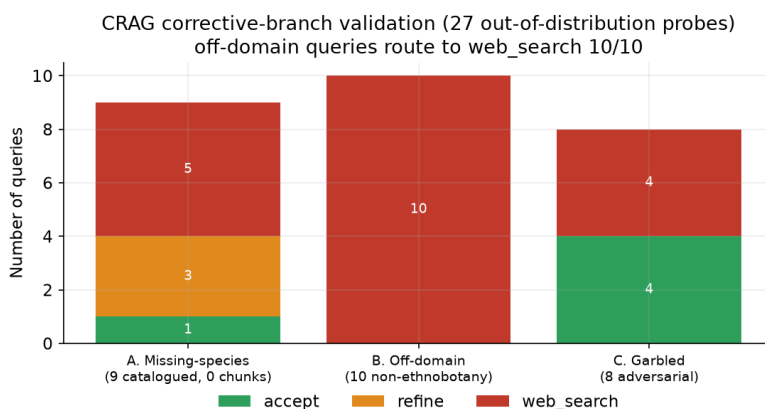
Figura 6. Validación de las ramas correctivas de CRAG sobre 27 consultas fuera de distribución.
