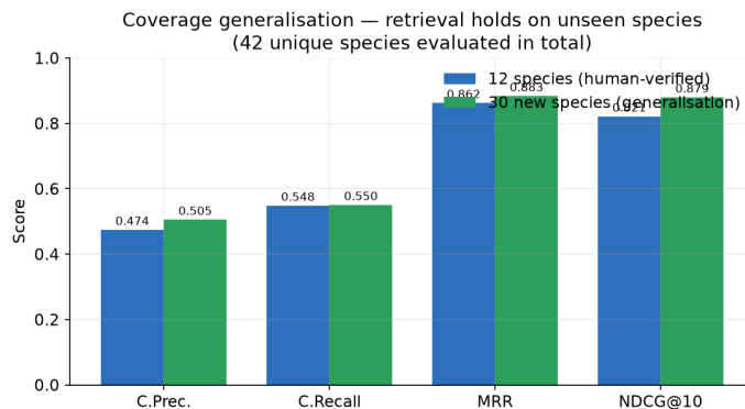
Figura 3. Generalización de la recuperación: la calidad se sostiene sobre 30 especies no vistas del corpus.
