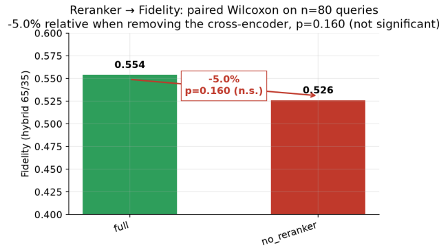
Figura 5. Fidelidad full vs. no_reranker : la dirección es consistente, pero la corrida final no alcanza significancia convencional ( p=0,160 ).
