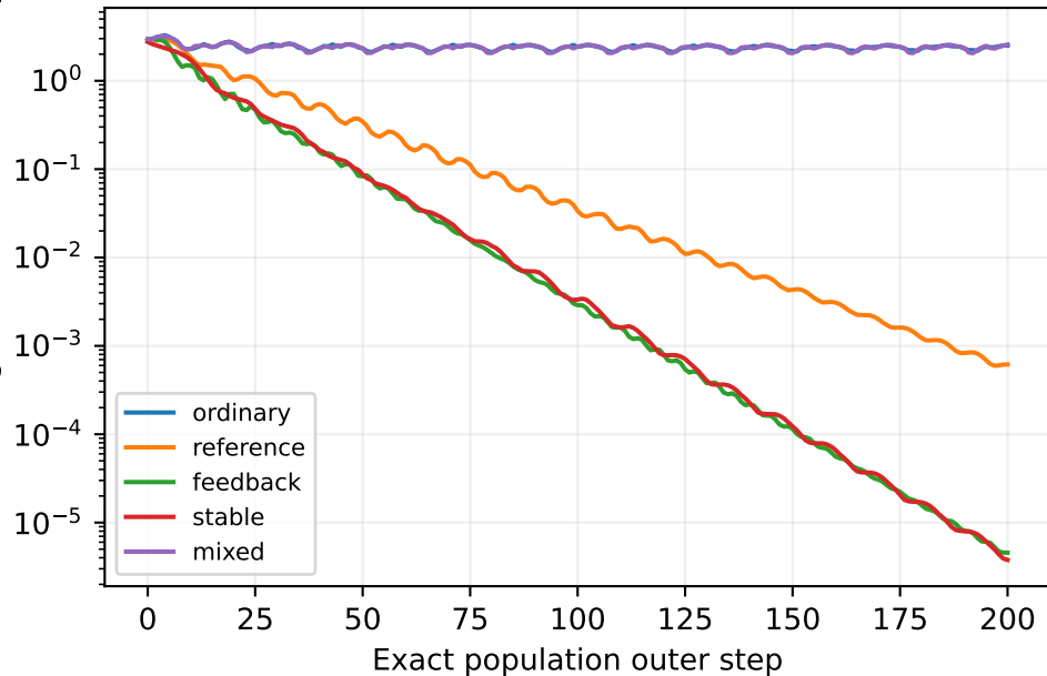
IPO
