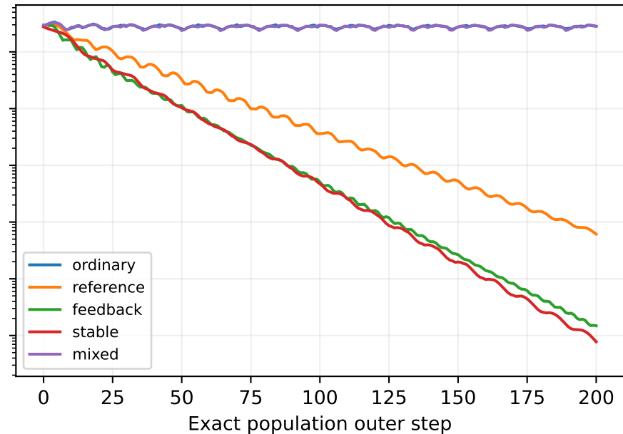
Actual DPO
