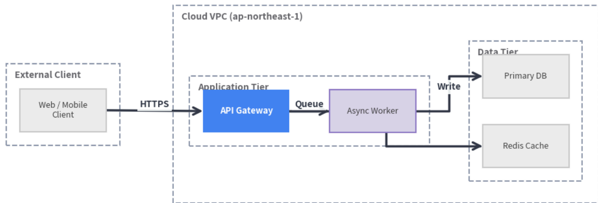
図 10.2: ArchitectureGraph による自動レイアウトとクラスタリング
