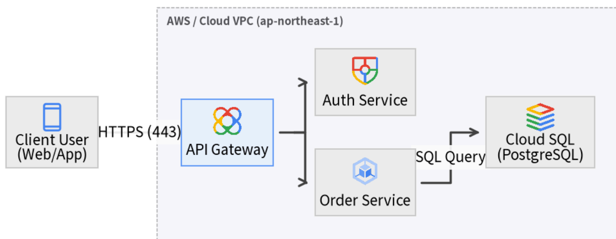
クラウドマイクロサービス構成図
