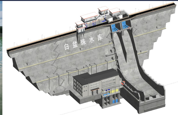
BIM效果
