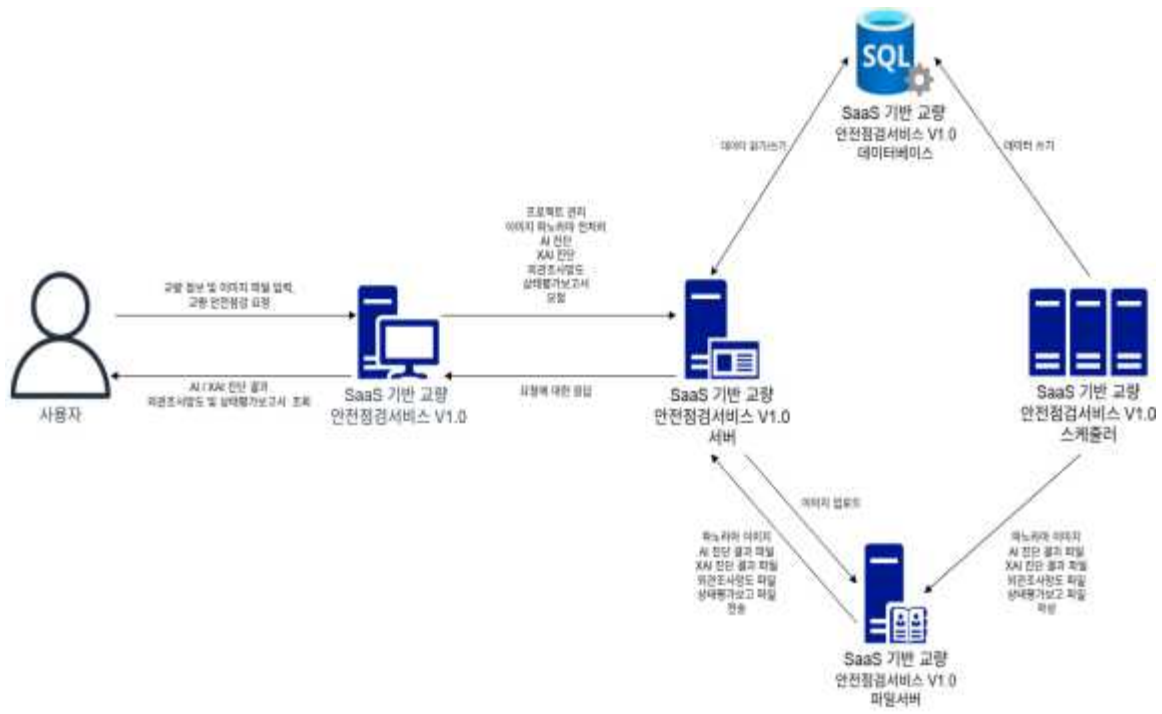
[그림 1] 교량 시설물 안전점검 자동화 웹서비스 V1.0 구성도
