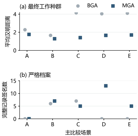
图 7 五个主场景的最终工作种群平均汉明距离与严格档案不重复完整记录签名数（描述性统计）
