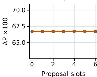
PTPC / dev.
