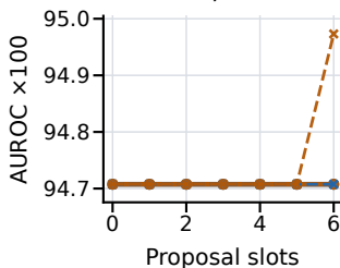
DTI / dev.
