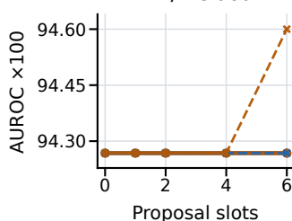
DTI / heldout
