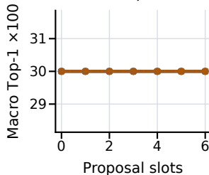
Tahoe / dev.
