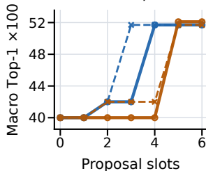
Norman / dev.
