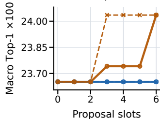
VCC / dev.
