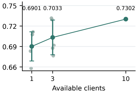
B AUROC
