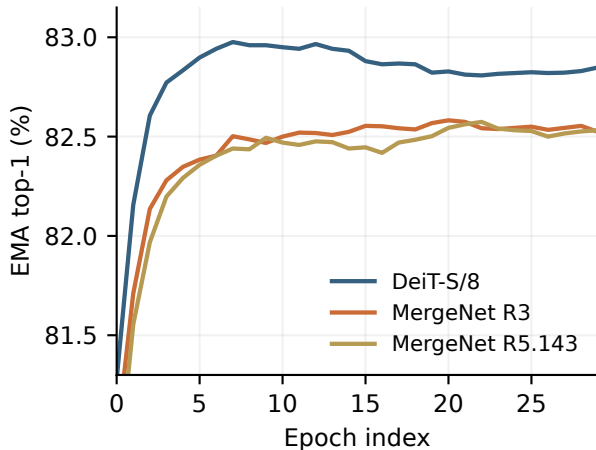
384 px: 30-epoch fine-tuning
