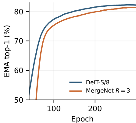
224 px, 300 epochs
