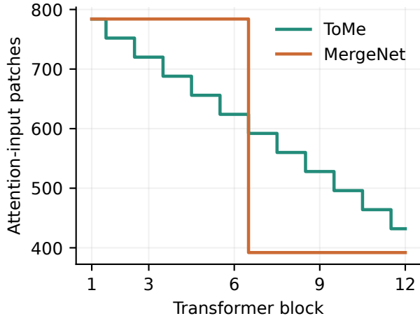
Layerwise token trajectories
