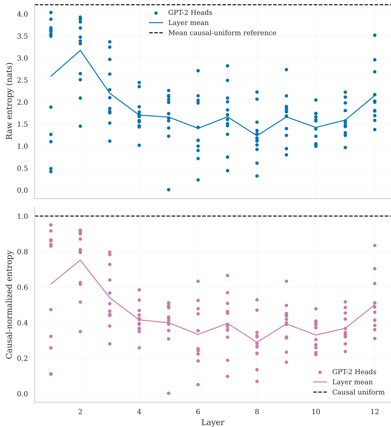
GPT-2 head entropy (N=158)
