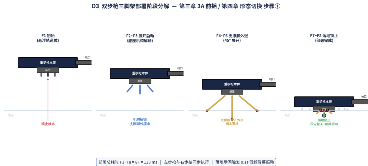
图 3-2 (D3) 三脚架部署 4 阶段分解 — F1 轨道位 → F2~F3 底座解锁 → F4~F6 三脚 45° 外张 → F7~F8 落地锁止（含灰尘粒子 + 低频振动）。单枪部署 8F = 133ms，双枪同步执行。同时适用于第四章形态切换步骤①。
