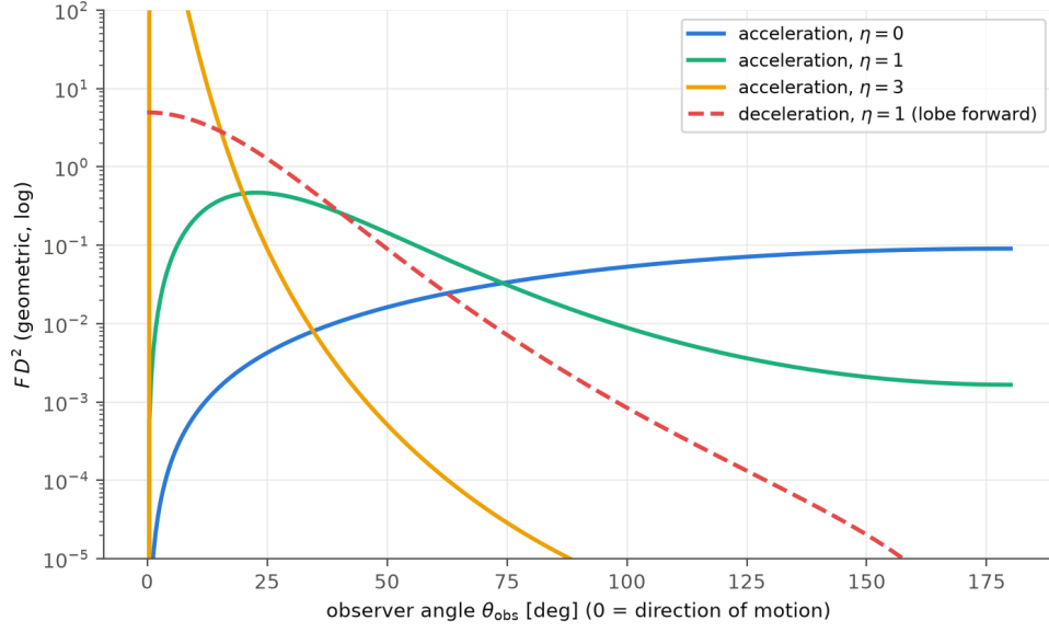
Figure 5: 数個のラピディティにおける飽和バーンの観測者系角度パターンと、減速バーンの反転ローブ。加速パターンの前方ヌルは厳密である。
