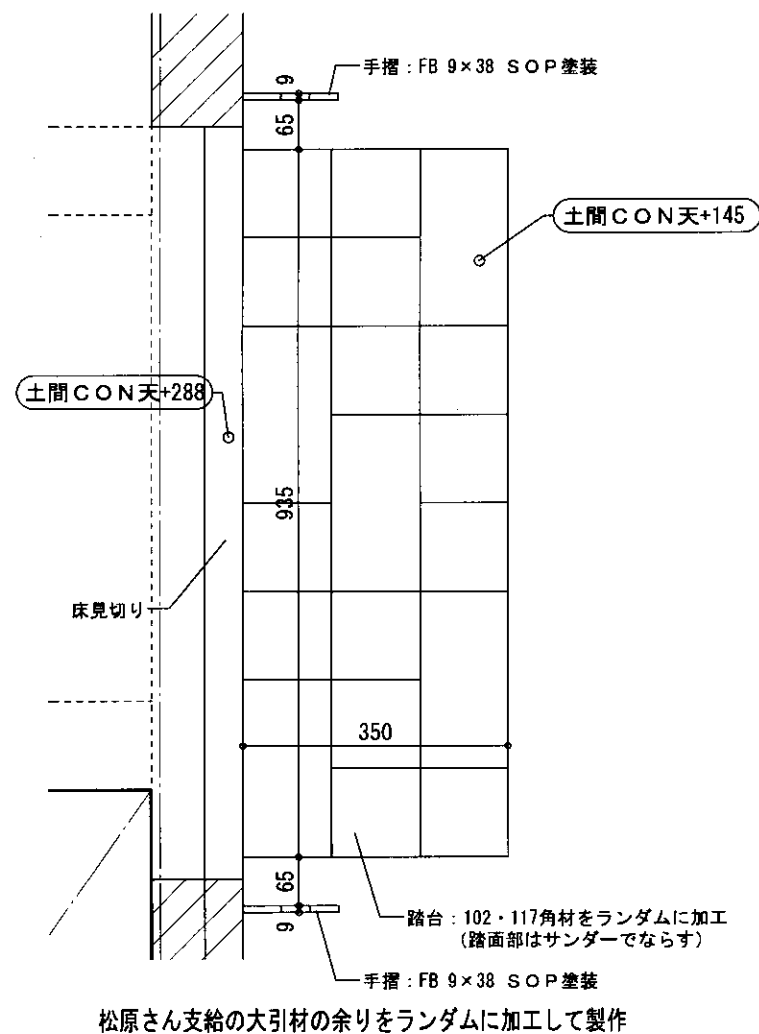
踏台詳細図 1/10
