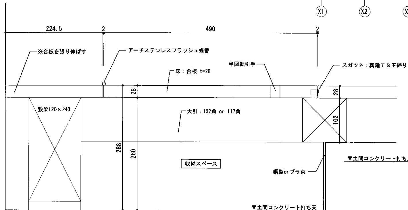
床下収納詳細図 1/5
