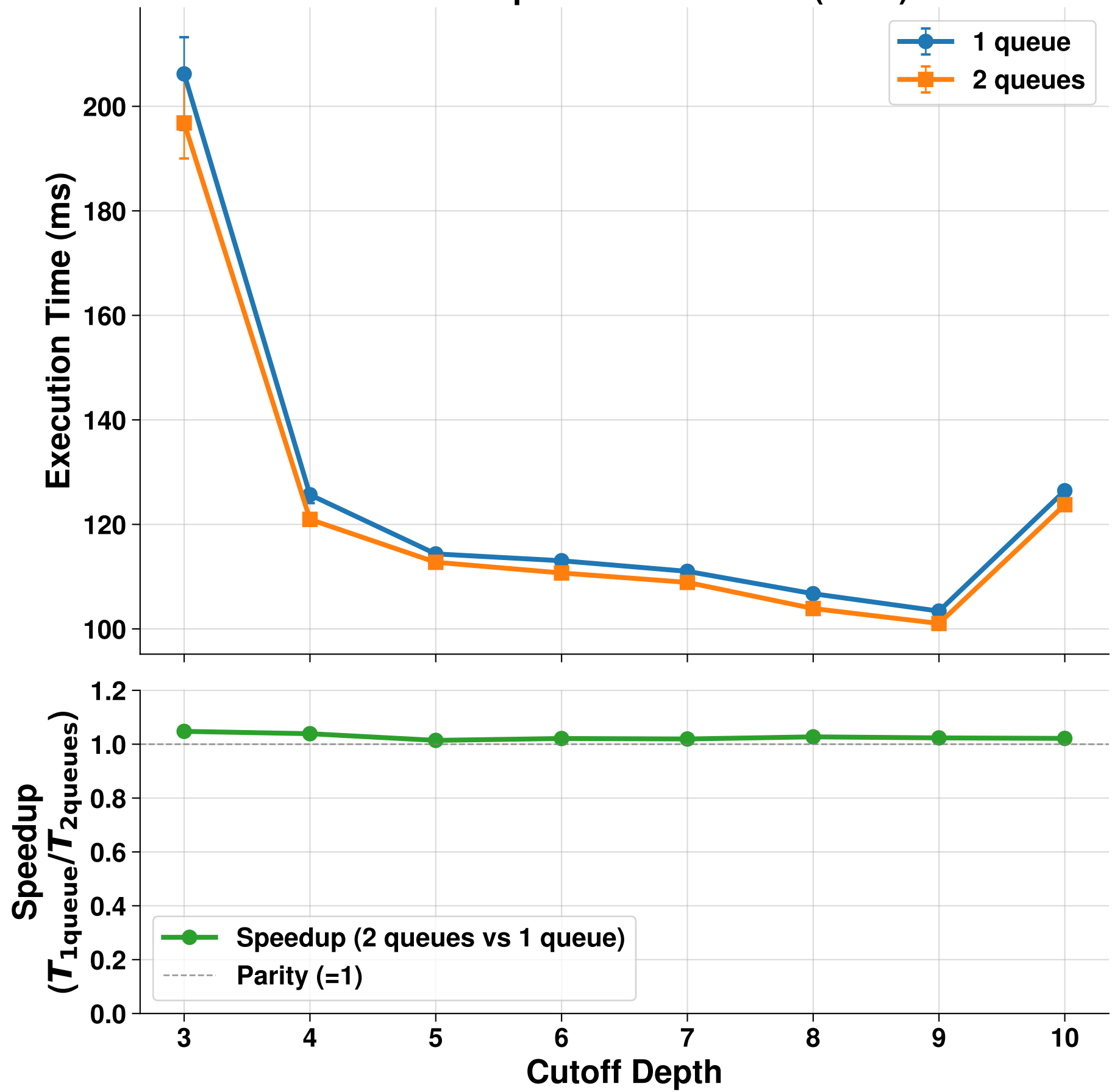
EPAQ Comparison: N-Queens (n=16)
