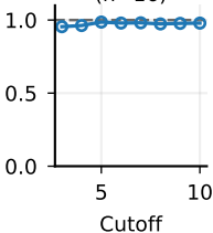
N-Queens ( n=16 )
