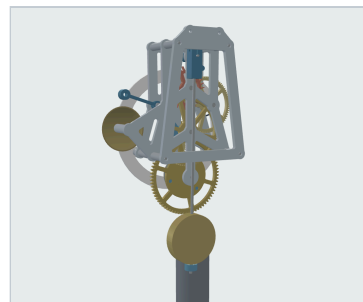
背面。壁フレームと、後ろ地板の裏の振り子。
