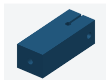
振り子ハンガー pendulum_hanger 16×41×14 mm 8.3 cm 3
