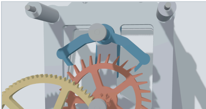
脱進機。アンクルとガンギ車の接触を計算して動かします。
