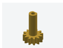
筒カナ 12枚 cannon_pinion 14×14×22 mm 0.9 cm 3
