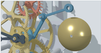
打鐘。ハンマーの尾が渦巻きカムに乗っています。
