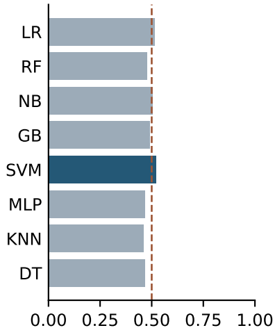
ROC-AUC
