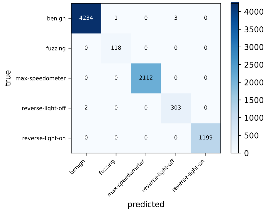
1D-CNN (macro-F1 0.997)
