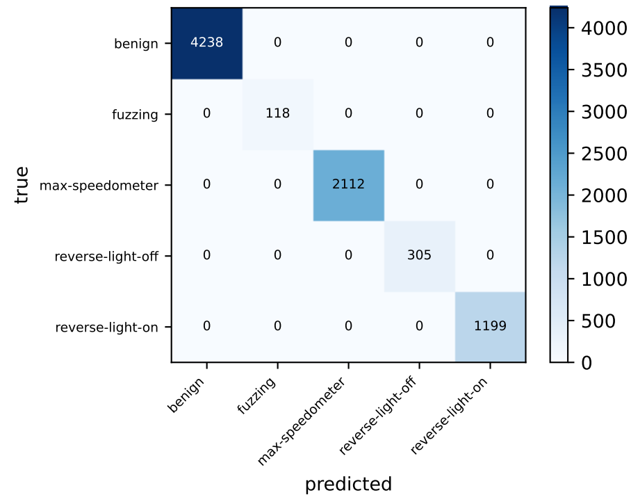
Random Forest (macro-F1 1.000)
