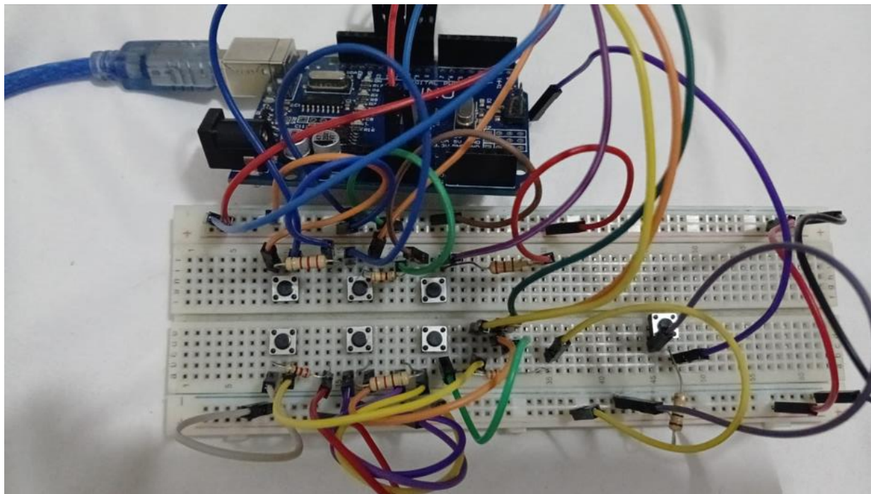
Figura 7 – Armado físico del circuito
