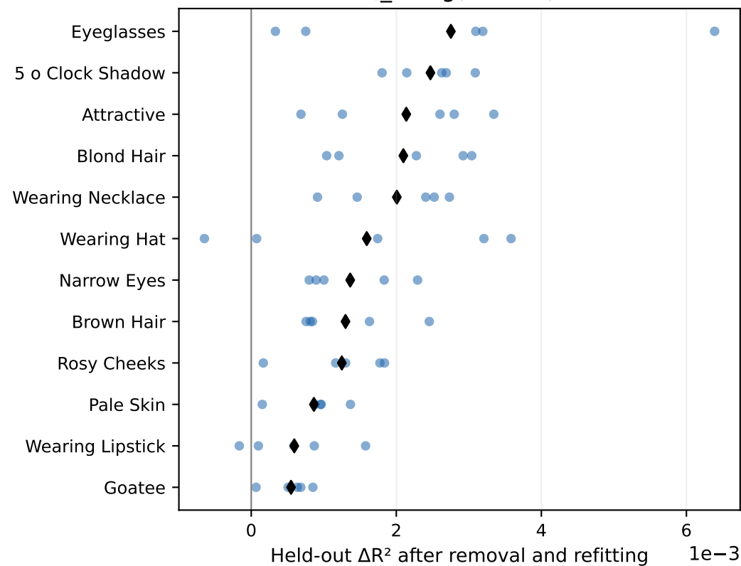
Q_u: log(2-RDR)
