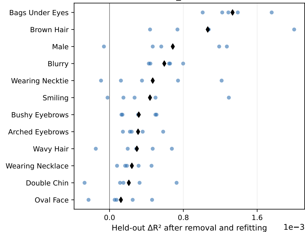
Q_u: RDR
