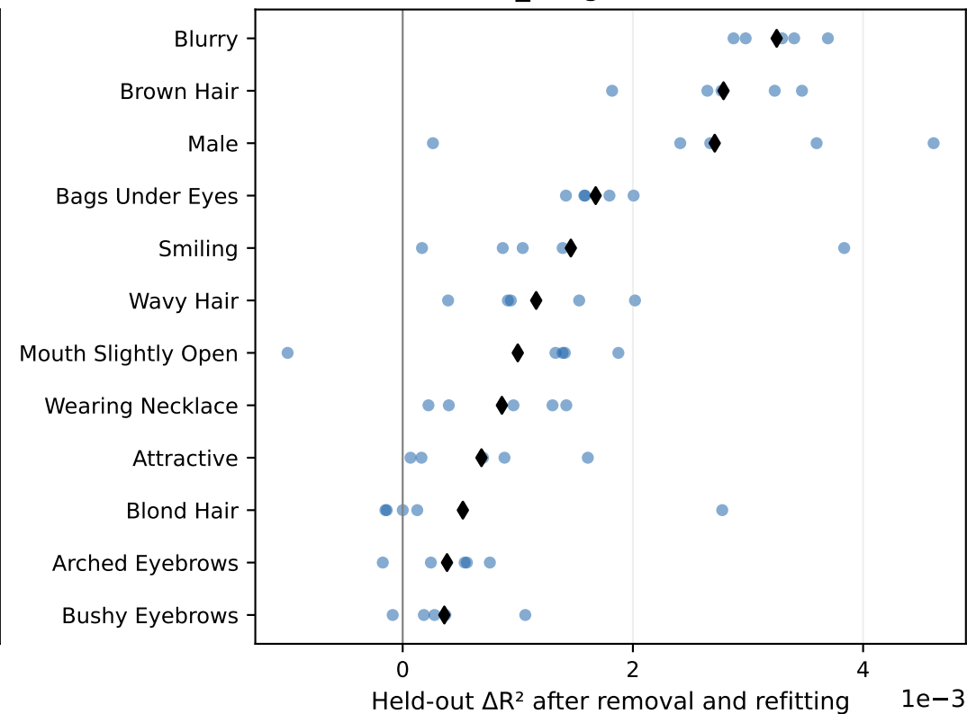
Q_u: log(2-RDR)
